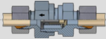
Rückschlagventile
