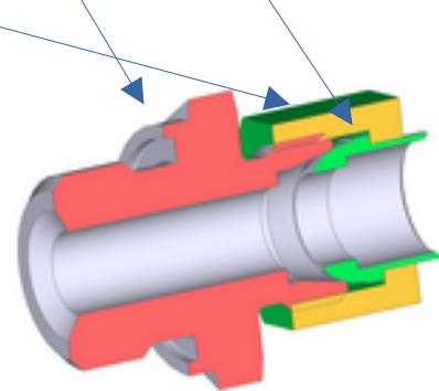
Schneidring Stutzen mit Kugelhülse und spez. Überwurfmutter
